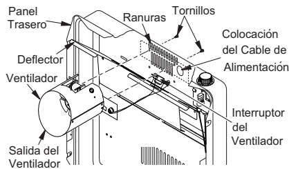
Figure 5: Frente del Calentador, Fijación del Ventilador
