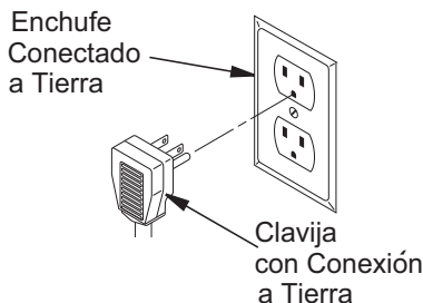
Figura 1: Clavija con conexión a tierra
