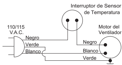
Figura 6 - Diagrama de Cableado para el Accesorio de Ventilador
