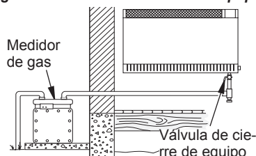
Figura 18 - Revisión de las uniones de gas para gas natural
