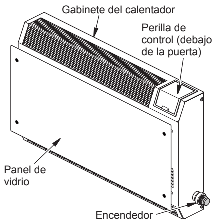
Figura 1 - Calentador de gas sin ventila-
