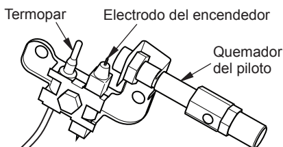
Figura 20 - Piloto (el piloto real puede ser distinto)
