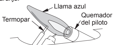
Figura 21 - Patrón correcto de la llama del piloto
