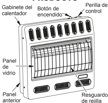
Figura 1 - Calentador de gas sin ventilación
