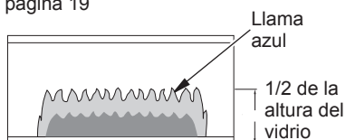
Figura 23 - Patrón correcto de la llama del quemador
