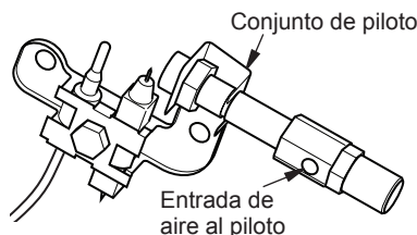
Figura 25 - Orificio de entrada de aire al piloto
