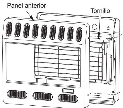
Figura 7 - Desmontaje del panel anterior del calentador
