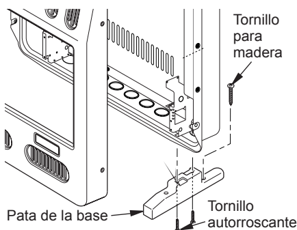
Figura 13 - Instalación de las patas de la base
