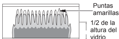
Figura 24 - Patrón incorrecto de la llama del quemador
