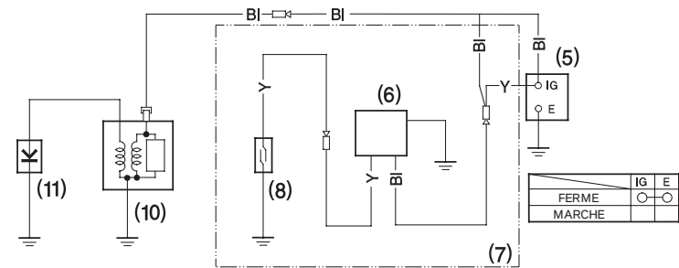
Avec système Oil Alert® et sans démarreur électrique
