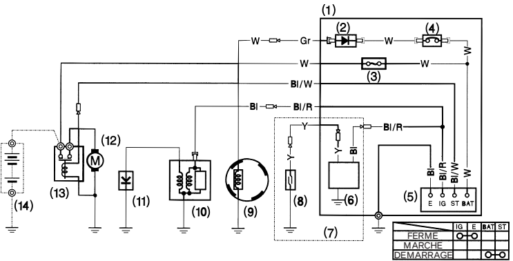
Avec système Oil Alert® et démarreur électrique
