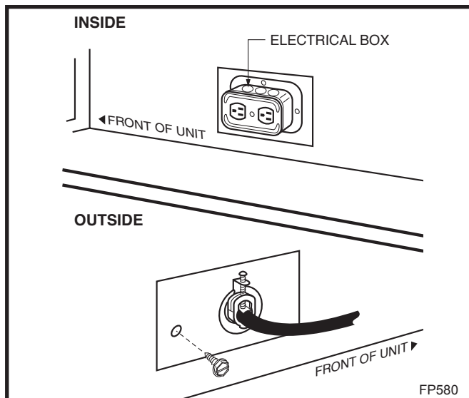
Fig. 9 EB-1 receptacle.
