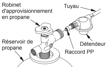
Figure 3 - Position du détendeur
