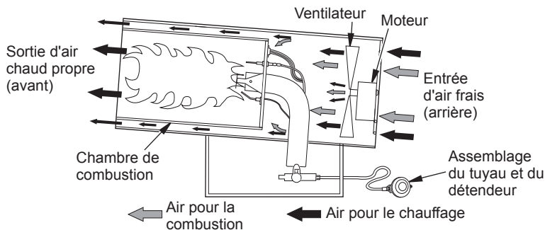
Figure 2 - Vue opérationnelle en coupe transversale
