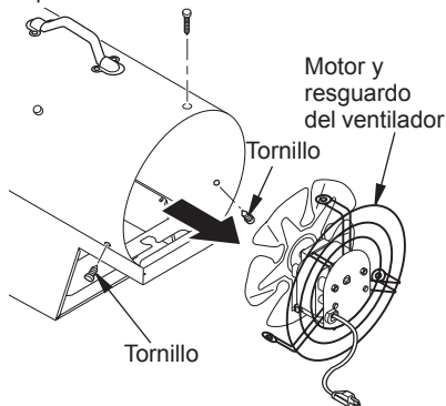
Figura 9 - Reemplazo del motor y el resguardo del ventilador en el calentador
