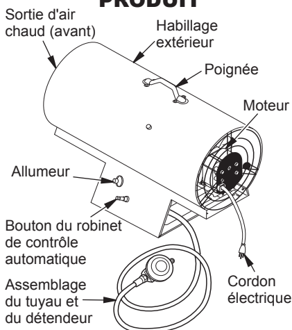
Figure 1 - Modèle à 35 000 BTU/H illustré
