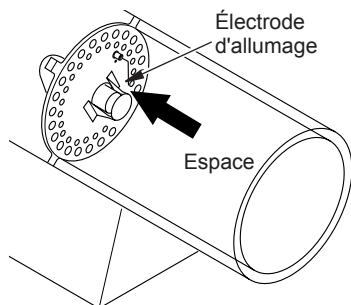
Figure 12 - Espace entre l'électrode d'allumage et la plaque
