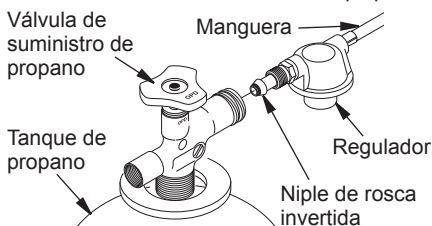
Figura 3 - Posición del regulador
