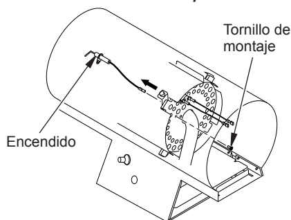
Figura 11 - Extracción del tornillo de montaje del encendido y el encendido
