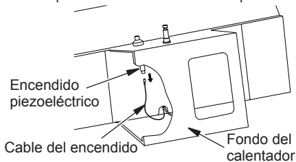
Figura 10 - Extracción del cable del encendedor del encendido piezoeléctrico
