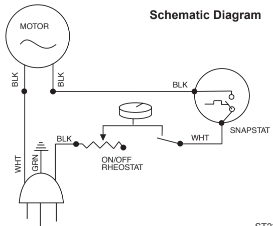
Fig. 41 Fan circuit.
