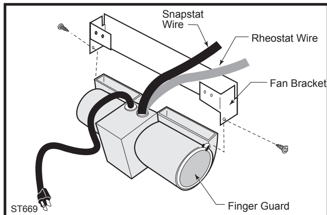
Fig. 8 Attach the fan assembly to the fan bracket.
