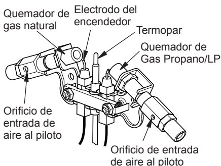
Figura 28 - Orificio de entrada de aire al piloto
