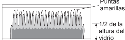
Figura 27 - Patrón incorrecto de la flama del quemador
