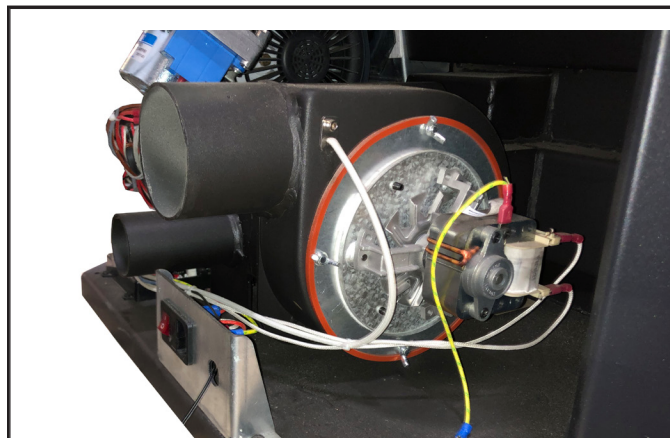
Figure 26 Ventilateur d'échappement du modèle H3W80XL
