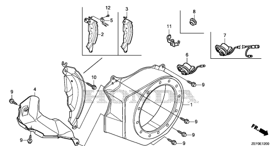
FAN COVER
