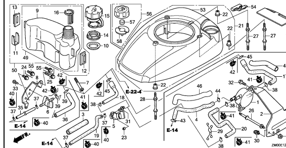
FAN COVER(2)
