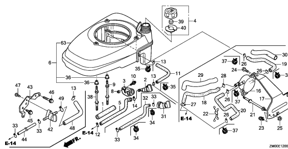
FAN COVER(1)
