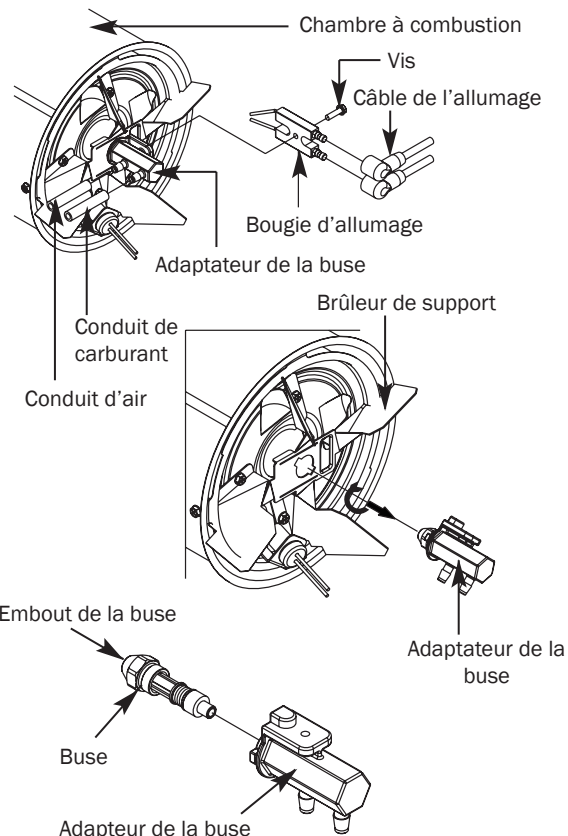
Figure 17 – Remplacement de la buse CP210FK
