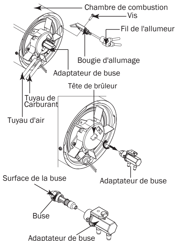
Figure 16 – Remplacement de la buse pour les modèles CP050EK-CP175FK
