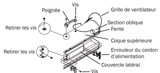
Figure 4 - Installation de la poignée et de l'enrouleur du cordon d'alimentation CP075EK
