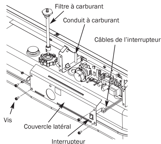
Figure 21 – Remplacement du filtre à carburant
