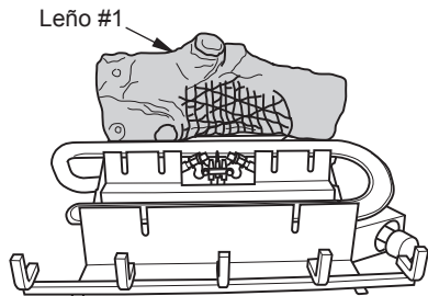
Figura 23 - Instalación Leño #1
