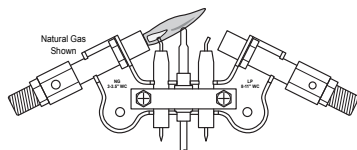
Figura 30 - Patrón correcto de la llama del piloto
