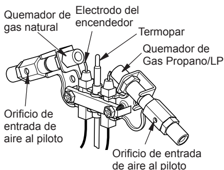
Figura 29 - Piloto
