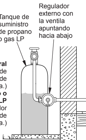
Figura 14 - Regulador externo con la ventila apuntando hacia abajo (sólo propano y gas LP)
