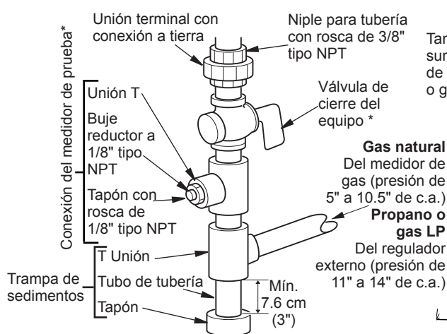
Figura 13 - Conexión de gas
