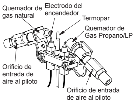
Figura 35 - Orificio de entrada de aire al piloto
