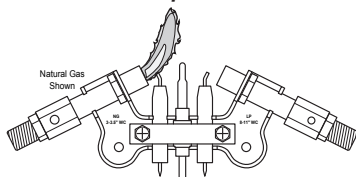
Figura 31 - Patrón incorrecto de la llama del piloto
