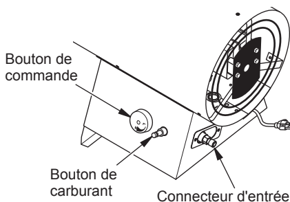
Figure 8 - Bouton de carburant et le bouton de commande de carburant (60 000 BTU/h Modèles)
