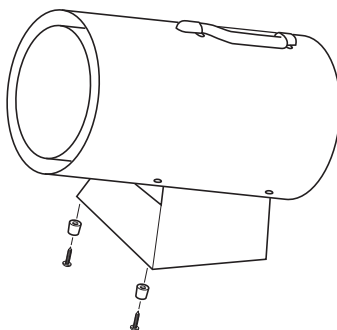
Figure 5 - Fixation de base Pieds Modèle PCFA40(-C)
