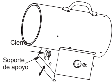
Figura 6 - Ajuste del Calentador Altura Modelo PCFA60V(-C)
