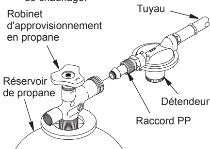
Figure 3 - Position du détendeur
