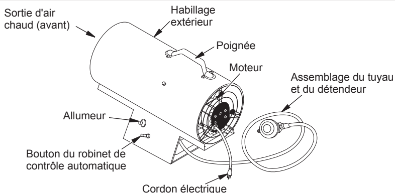
Figure 1 - Modèle à 40 000 BTU/H illustré
