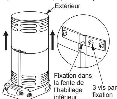
Figure 2 - Soulèvement de l'habillage extérieur
