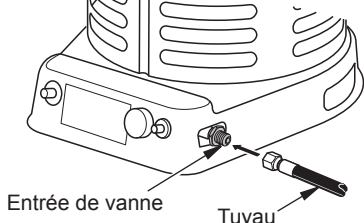
Figure 4 - Tuyau et entrée de vanne
