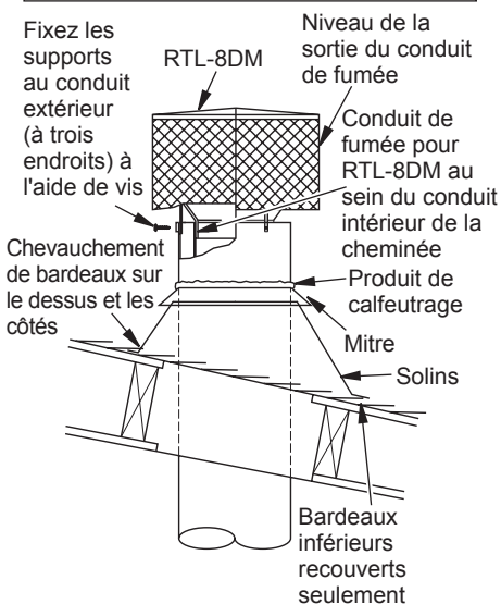
Figure 17 - Terminaison
