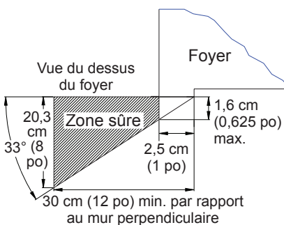
Figure 5 - Dégagement du manteau de foyer latéral
