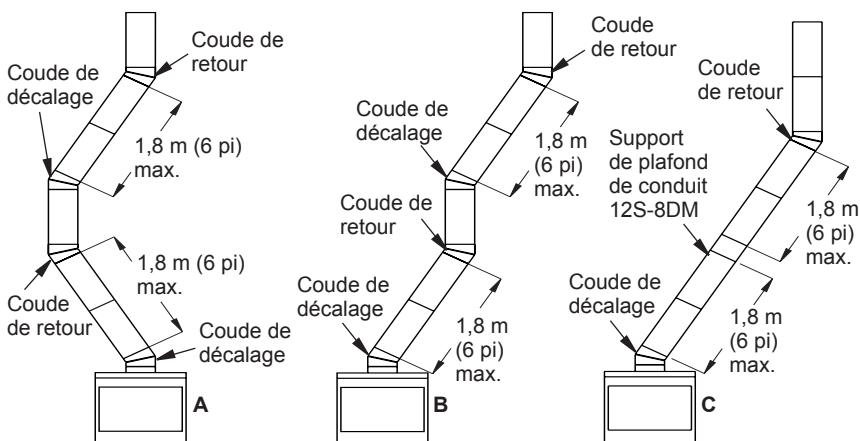
Figure 9 - Installation représentative d'un décalage
