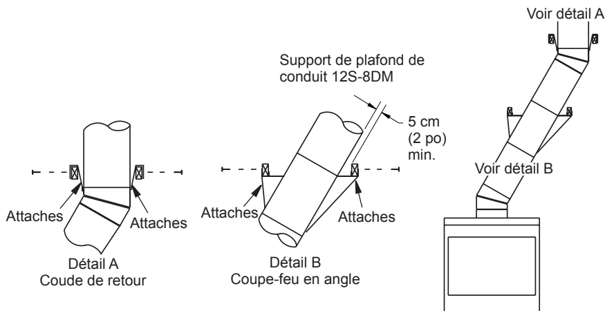
Figure 10 - Conduit de support de plafond 12S-8DM
