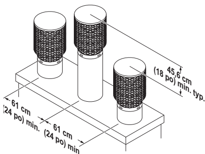
Figure 18 - Installation avec plusieurs enchâssures
