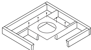
Figure 13 - Entretoise de pare-feu dans le cas d'un grenier au-dessus d'un plafond
