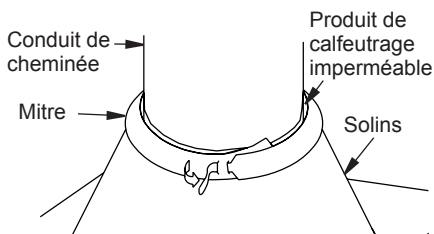
Figure 16 - Mitre
