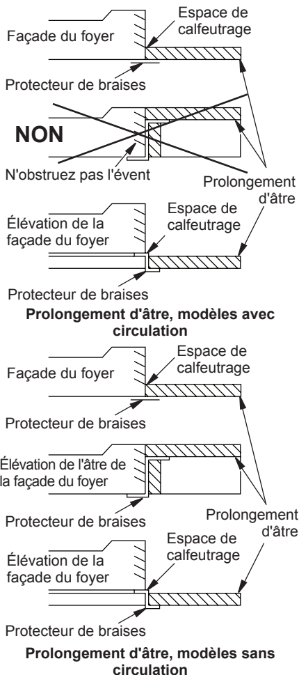
Figure 3 - Prolongement d'âtre
