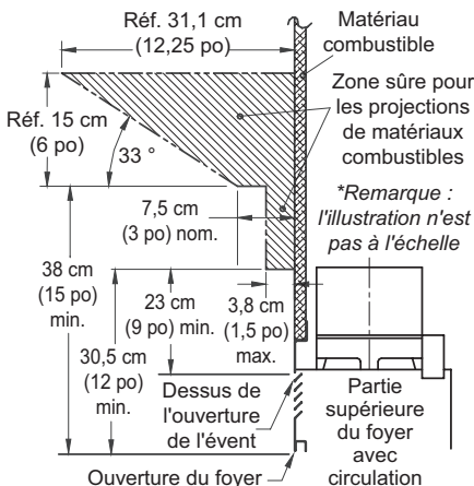
Figure 4 - Dégagements du manteau de foyer par rapport aux matériaux combustibles
