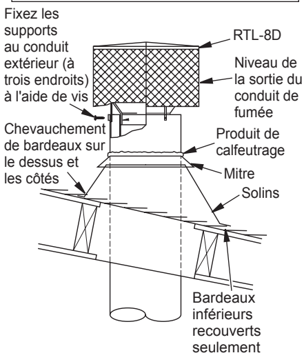
Figure 17 - Terminaison
