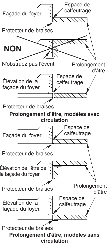
Figure 3 - Prolongement d'âtre
