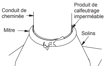
Figure 16 - Mitre
