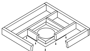
Figure 13 - Entretoise de pare-feu dans le cas d'un espace habitable au-dessus d'un plafond
