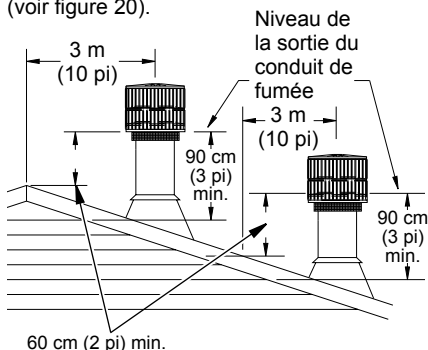
Figure 20 - Règle de 3 m (10 pi)
