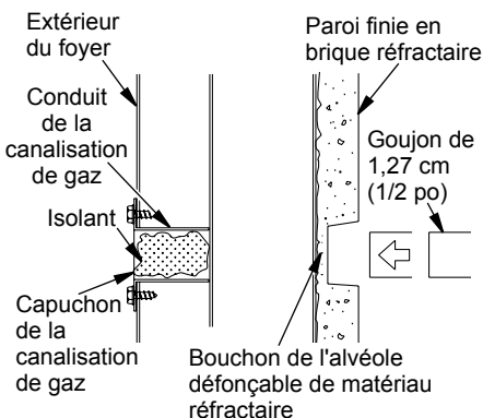
Figure 22 - Alvéole défonçable de la canalisation de gaz
