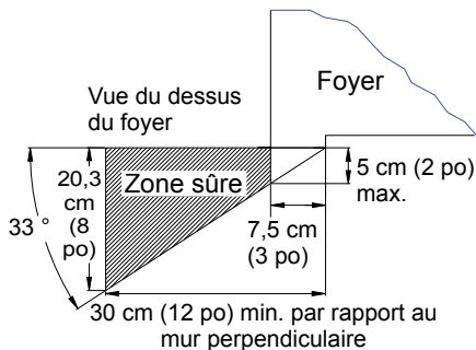
Figure 6 - Dégagement du manteau de foyer latéral
