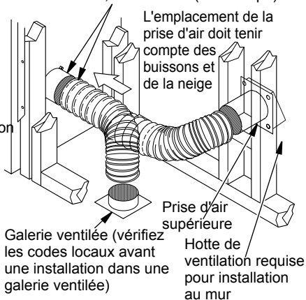
Figure 8 - Prêt-à-monter de gaine d'air extérieur
