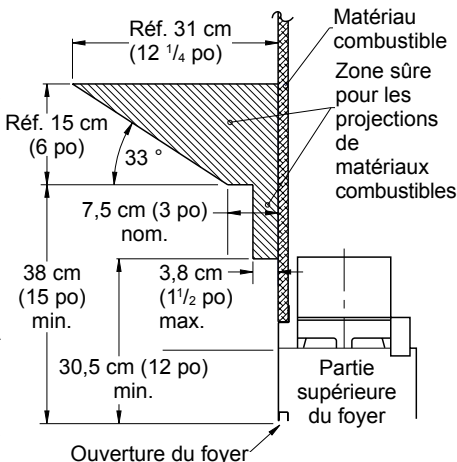
Figure 5 - Dégagements du manteau de foyer par rapport aux matériaux combustibles (sans événement)
