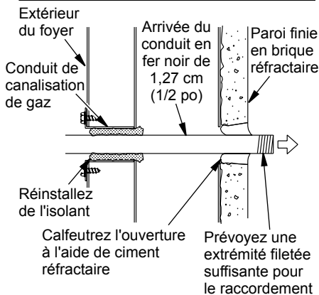
Figure 23 - Installation de la canalisation de gaz
