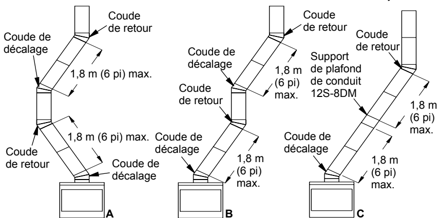
Figure 10 - Installation représentative d'un décalage
