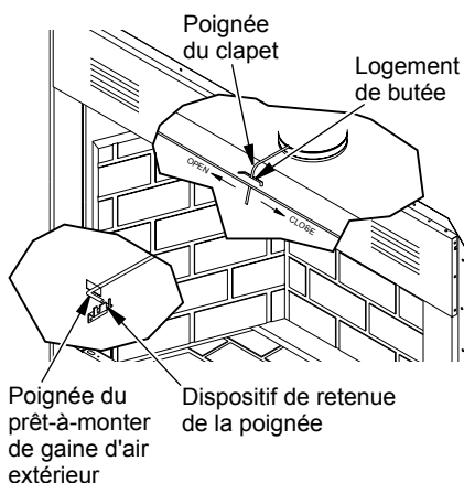
Figure 25 - Poignets du clapet et du prêt-à-monter de gainé d'air extérieur
