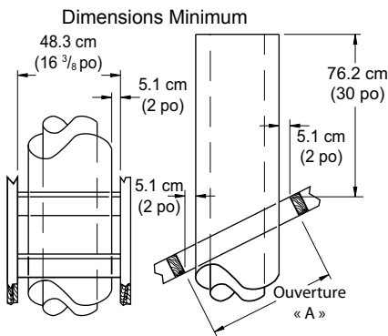
Figure 13 - Entretoise de pare-feu dans le cas d'un espace habitable au-dessus d'un plafond
