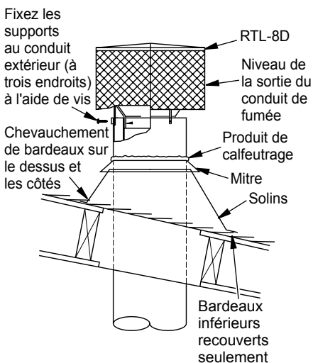
Figure 18 - Terminaison
