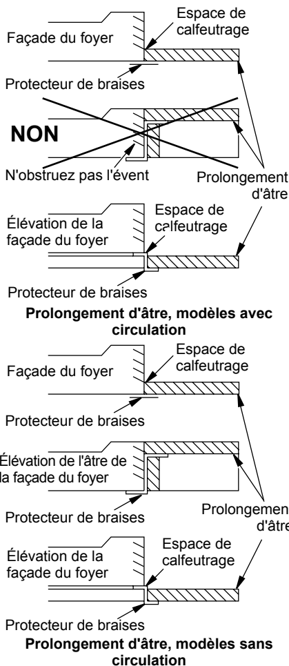
Figure 3 - Prolongement d'âtre
