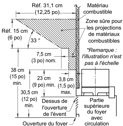
Figure 4 - Dégagements du manteau de foyer par rapport aux matériaux combustibles (avec événement)
