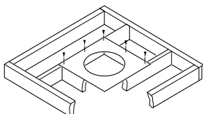
Figure 14 - Entretoise de pare-feu dans le cas d'un grenier au-dessus d'un plafond
