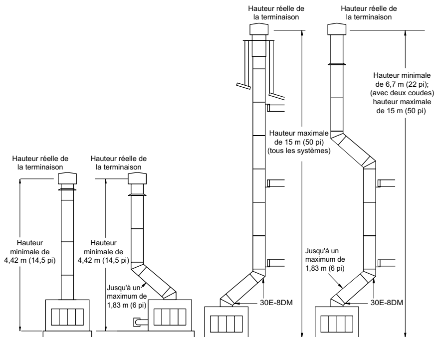
Figure 21 - Installations résidentielles représentatives
