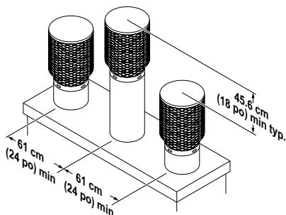
Figure 19 - Installation avec plusieurs enchâssures
