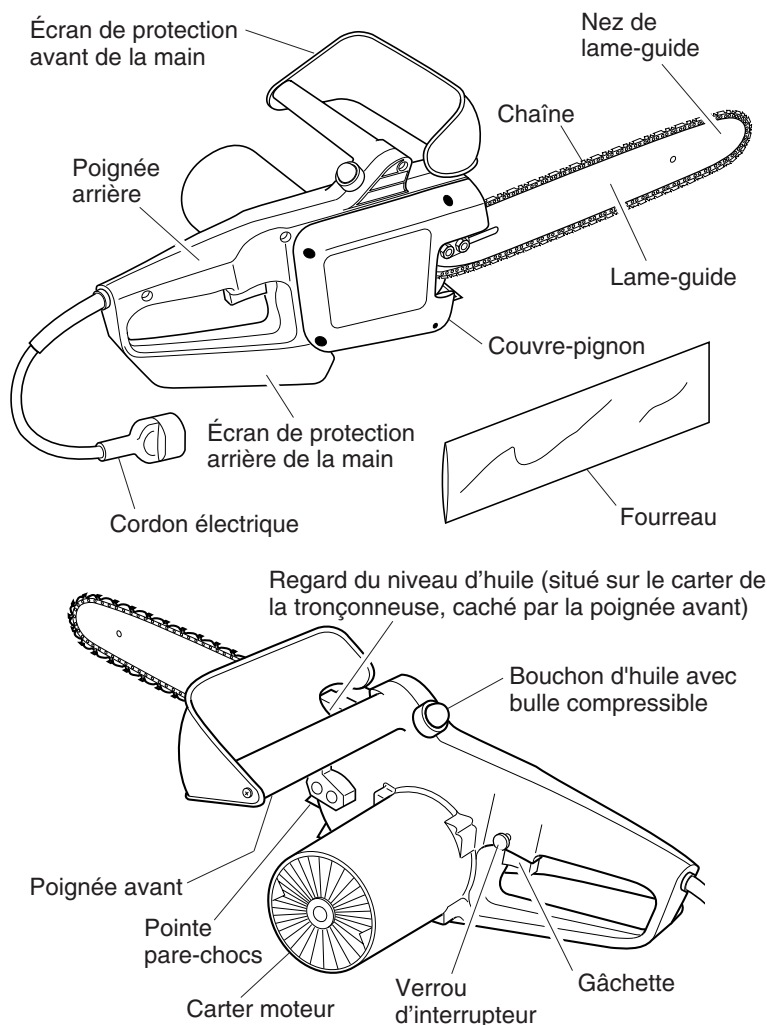
Figure 2 - Tronçonneuse électrique
