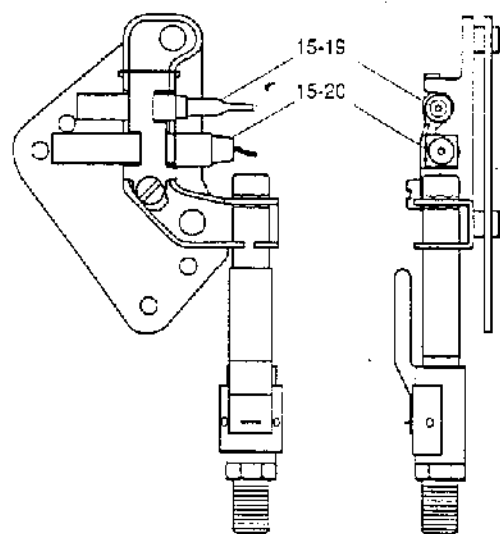
ODS/PILOT ASSEMBLY
