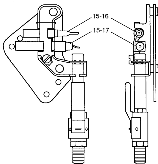
ODS/PILOT ASSEMBLY
