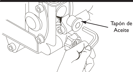
Figura 41 - Cambio del Aceite de la Bomba
