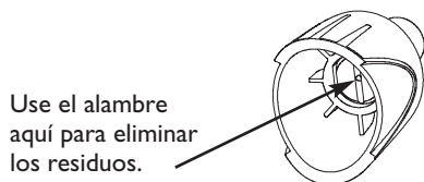
Figura 39 - Mantenimiento de la Boquilla
