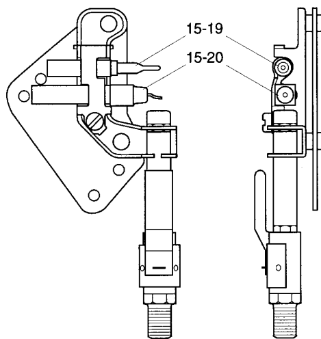
ODS/PILOT ASSEMBLY
